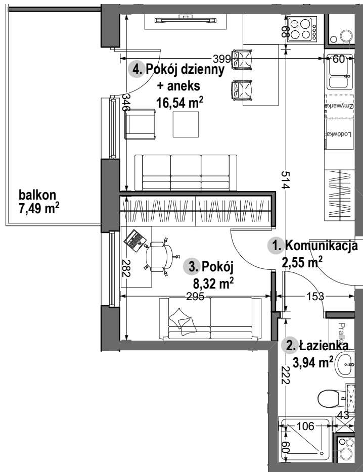
BUDYNEK NR 2
