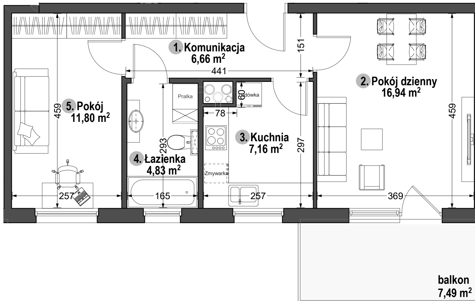
BUDYNEK NR 1
