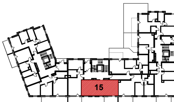
BUDYNEK NR 1
