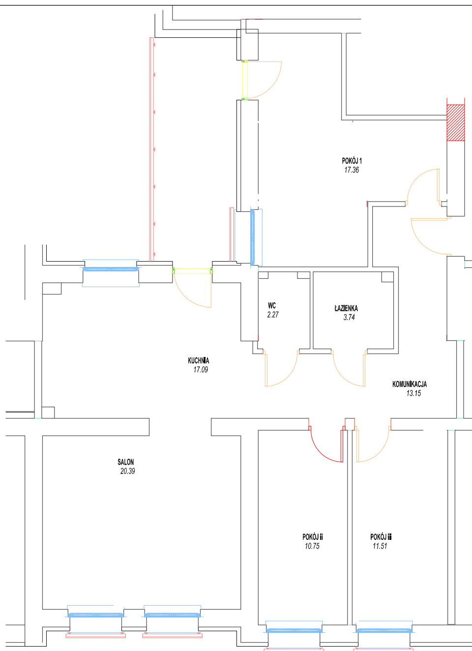
Rzut I PIĘTRA budynku z zaznaczeniem położenia lokalu mieszkalnego
